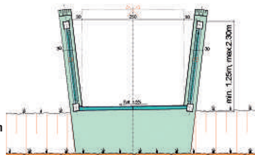
Die Konstruktion im Quer- und Längsschnitt.
